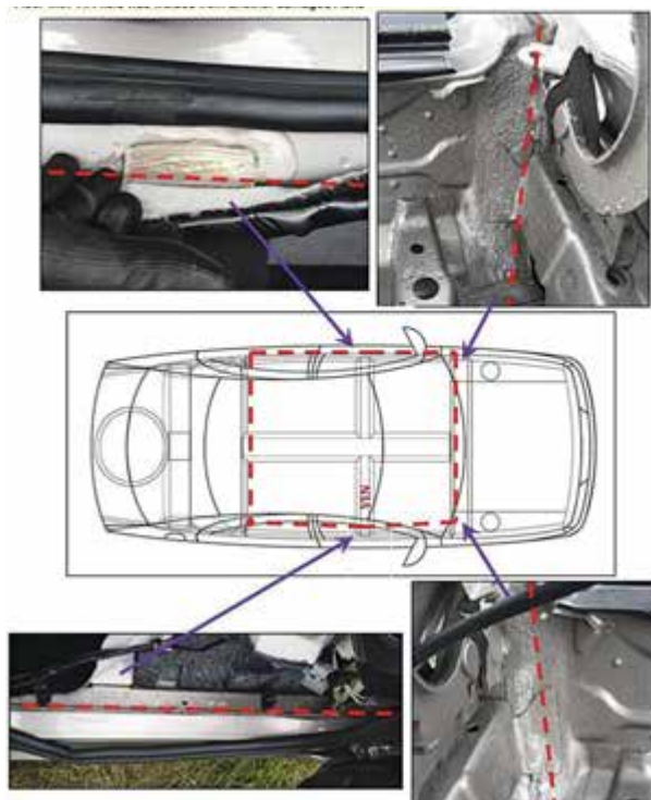
Przykład sfalszowanego oznaczenia identyfikacyjnego przez wspawanie do pojazdu elementu podłogi z numerem identyfikacyjnym VIN pochodzącym z innego pojazdu
