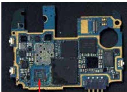
Miejsce po wylutowaniu kości pamięci z widocznymi śladami oderwanych pinów
